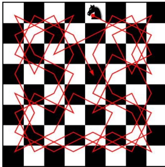
Abbildung 4.2: Das Rösselsprungproblem
